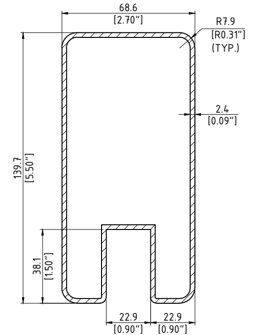
SECTION - TYPICAL CROSS SECTION SCALE: N.T.S.
