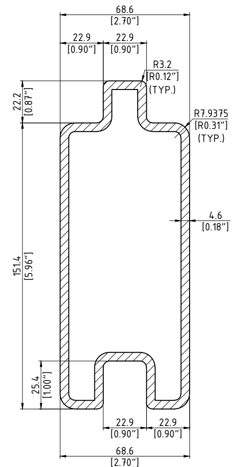
SECTION - TYPICAL CROSS SECTION SCALE: N.T.S.
