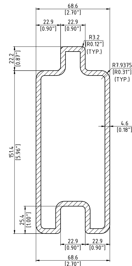
A SECTION - TYPICAL CROSS SECTION SCALE: N.T.S.
