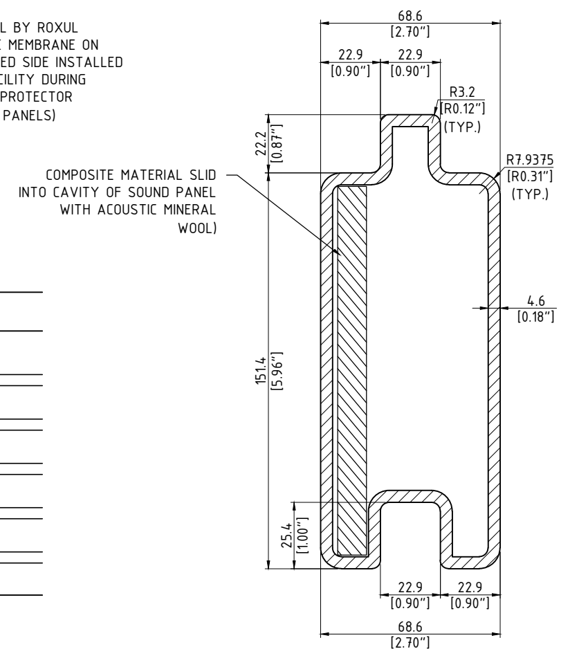
A SECTION - TYPICAL CROSS SECTION SCALE: N.T.S.
