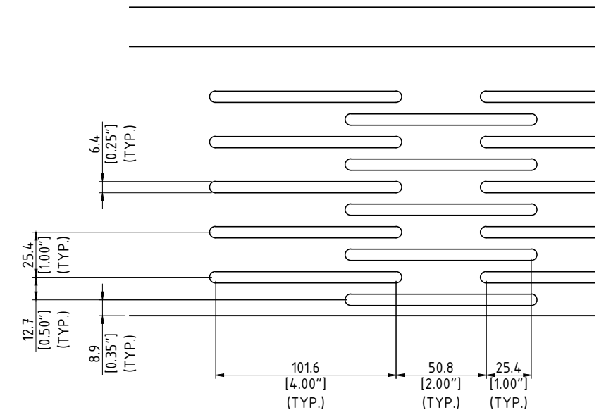
1 SW-025 DETAIL - ROUTING PATTERN SCALE: N.T.S.
