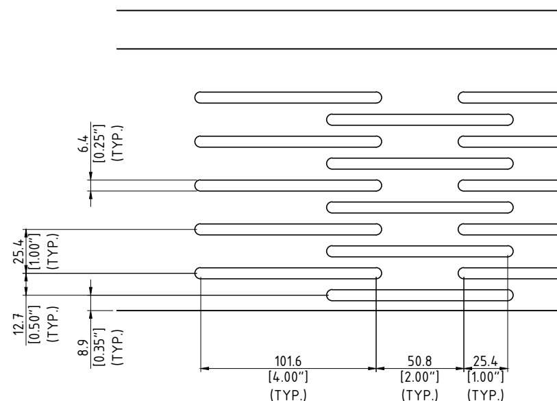
1 SW-020 DETAIL - ROUTING PATTERN SCALE: N.T.S.
