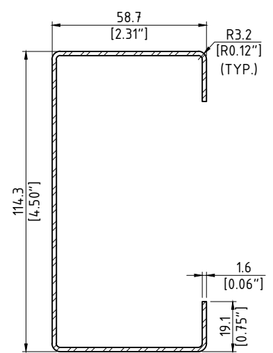
SECTION - TYPICAL CROSS SECTION SCALE: N.T.S.
