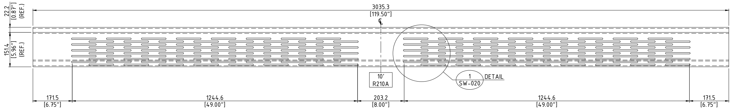
SILENT PROTECTOR ROUTING PATTERN R210A - 3.035 m [119.5"] SECTION SCALE: N.T.S.
