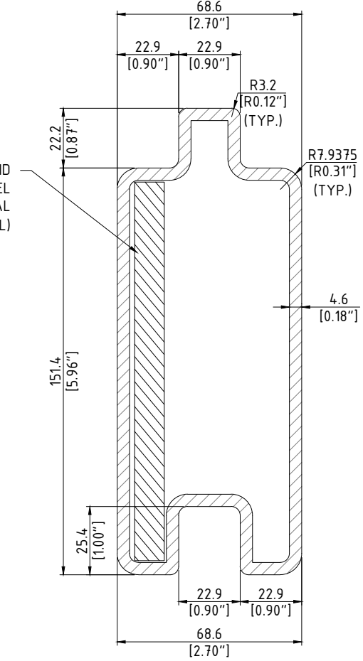
A SW-025 SECTION - TYPICAL CROSS SECTION SCALE: N.T.S.
