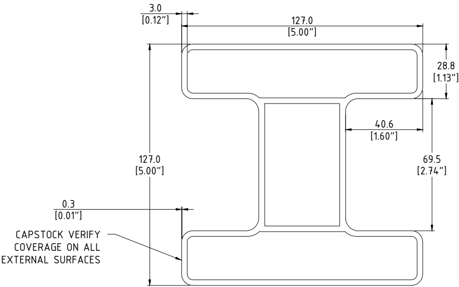
A SW-025 SECTION - TYPICAL CROSS SECTION SCALE: N.T.S.
