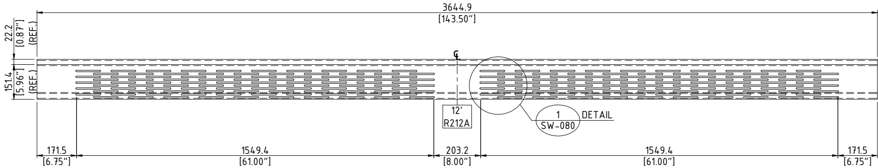
SILENT PROTECTOR XL ROUTING PATTERN R212A - 3.645 m [143.5"] SECTION SCALE: N.T.S.
