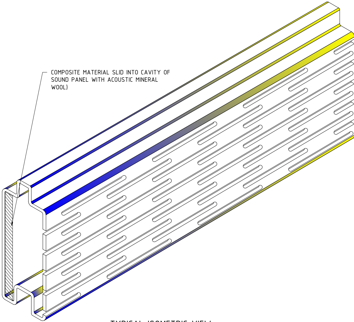
TYPICAL ISOMETRIC VIEW SCALE: N.T.S.
