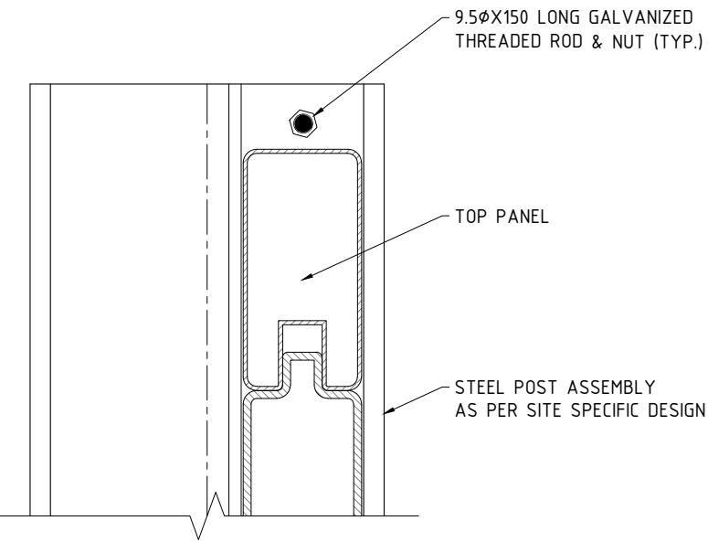
SECTION - SIDE VIEW SCALE: N.T.S.
