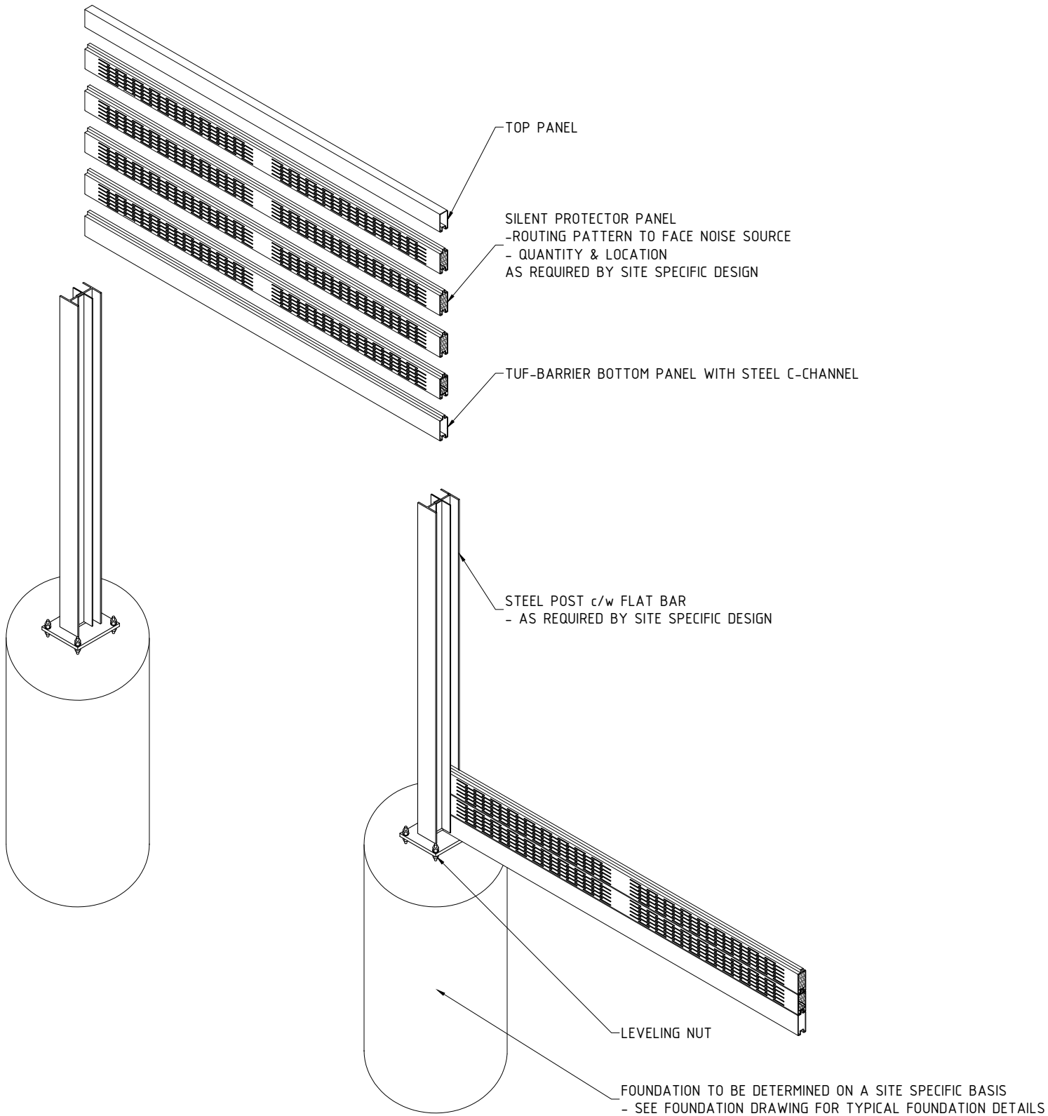
TYPICAL ASSEMBLY ISOMETRIC DETAIL SCALE: N.T.S.
