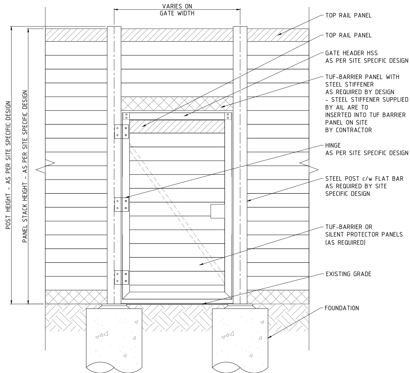
TYPICAL GATE ASSEMBLY ELEVATION SCALE: N.T.S.
