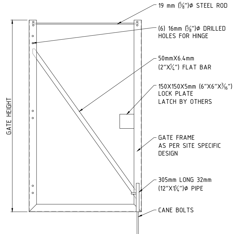
TYPICAL LEFT GATE DETAIL SCALE: N.T.S.
