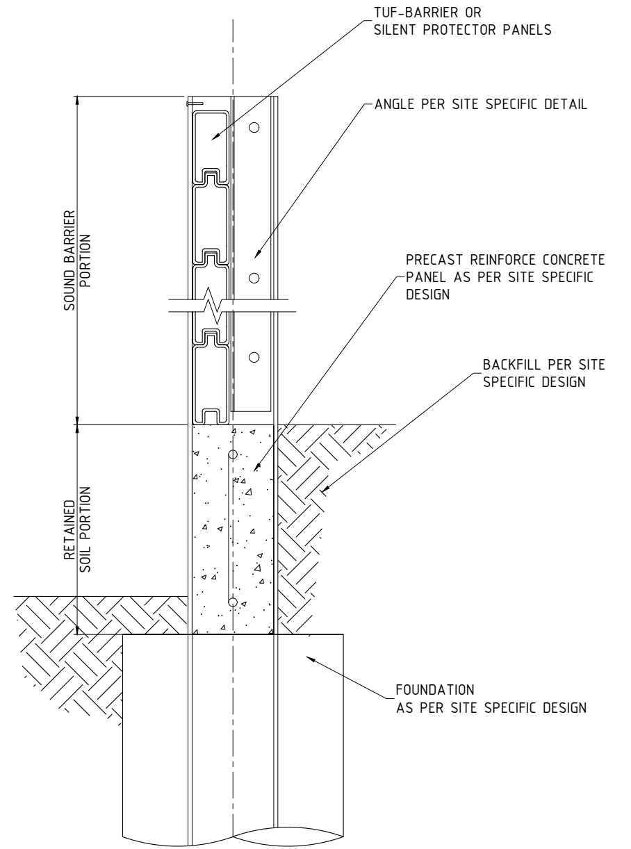
SECTION - TYPICAL ANGLE CROSS SECTION SCALE: N.T.S.
