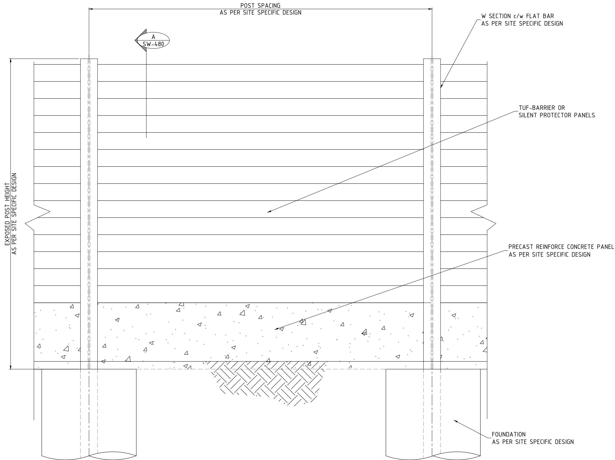
TYPICAL ELEVATION VIEW SCALE: N.T.S.
