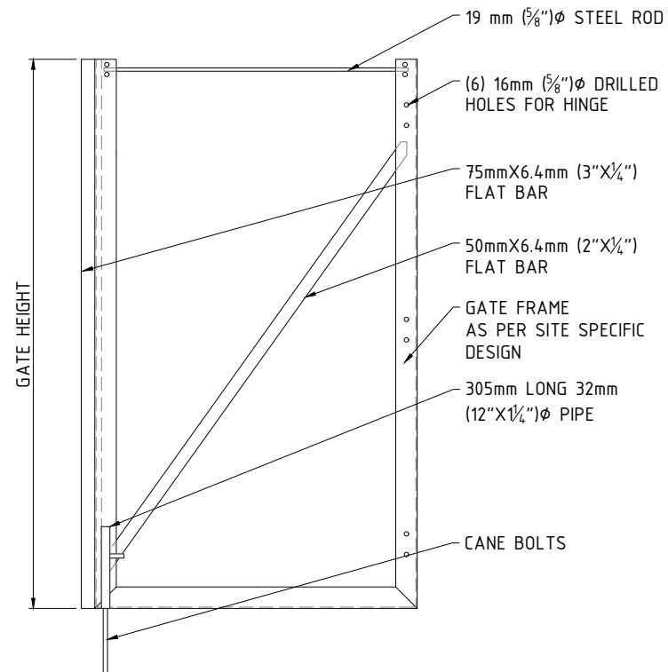
TYPICAL RIGHT GATE DETAIL SCALE: N.T.S.
