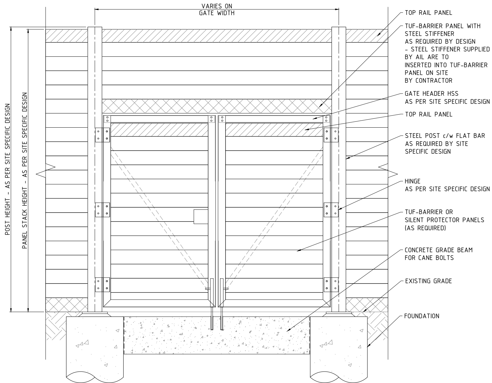
TYPICAL GATE ASSEMBLY ELEVATION SCALE: N.T.S.
