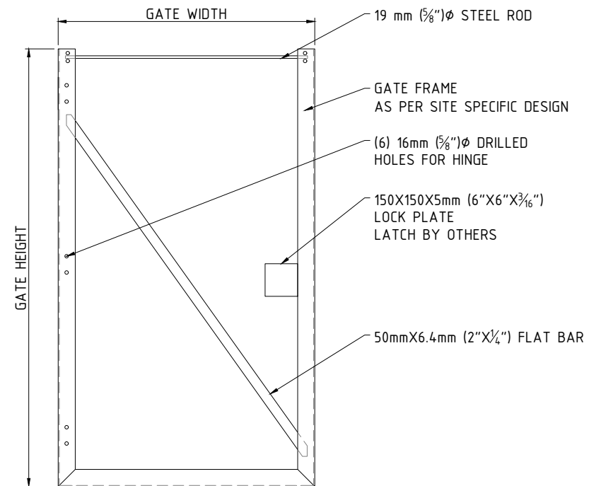
TYPICAL GATE FRAME DETAIL SCALE: N.T.S.
